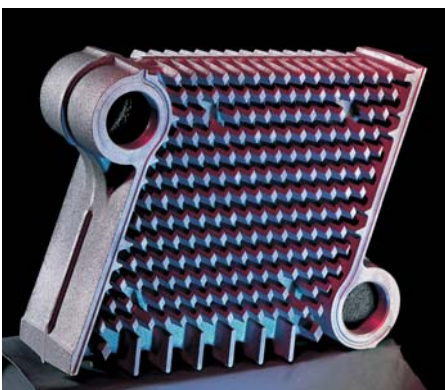
Výchřivé plochy ze speciální šedé litiny s lamelovým grafitem.
